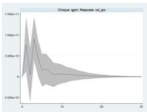
Figura 2: Função de resposta ao impulso do volume arrecadado nos IPOs
