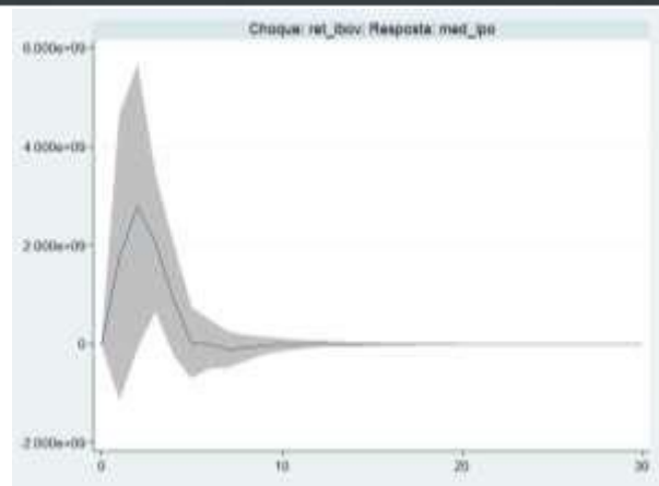
Figura 7: Função de resposta ao impulso da média arrecadada nos IPOs
