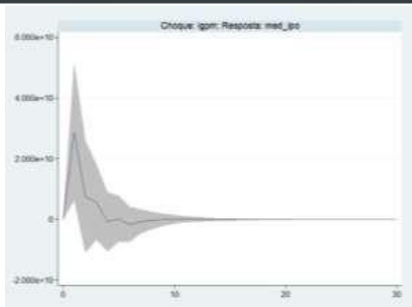
Figura 6: Função de resposta ao impulso da média arrecadada nos IPOs
