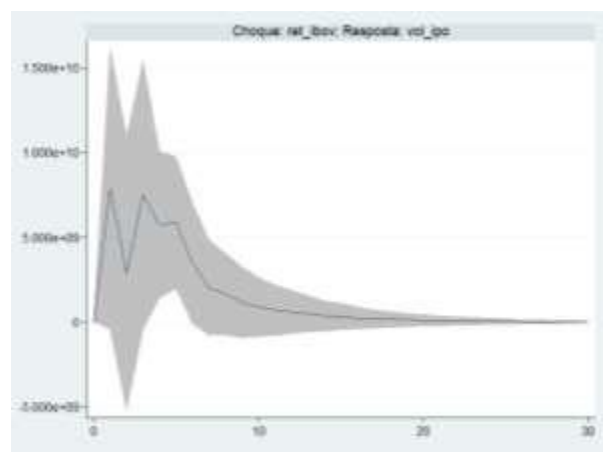
Figura 3: Função de resposta ao impulso do volume arrecadado nos IPOs
