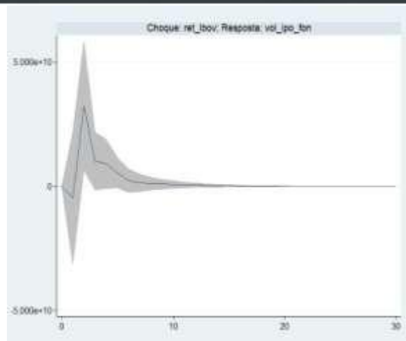
Figura 5: Função de resposta ao impulso do volume arrecadado nos IPOs e Follow-ons
