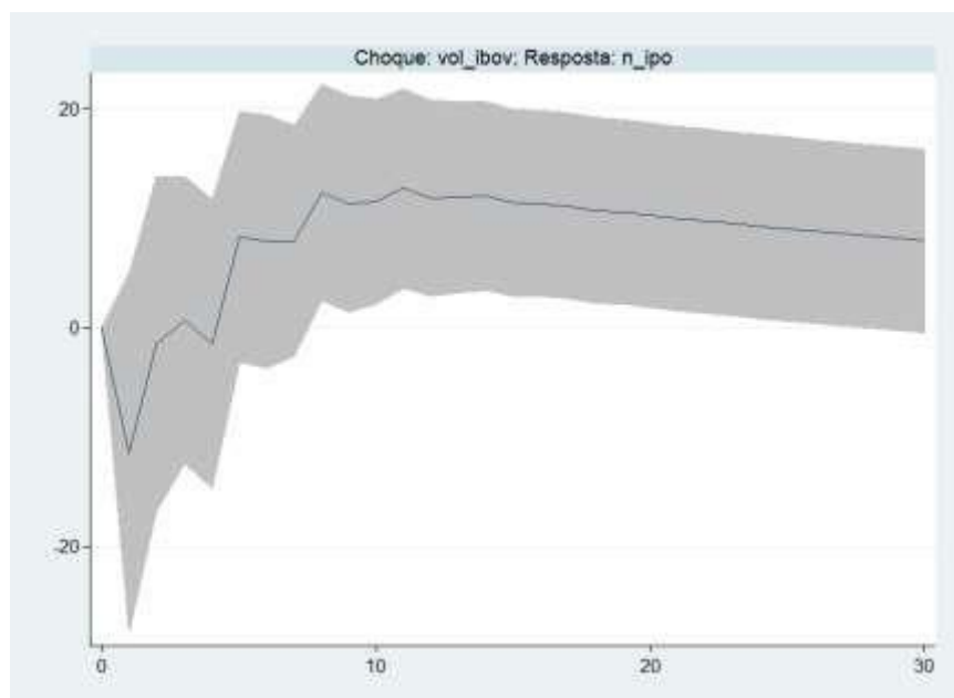
Figura 1: Função de resposta ao impulso do número de IPOs
