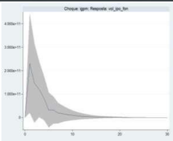
Figura 4: Função de resposta ao impulso do volume arrecadado nos IPOs e Follow-ons
